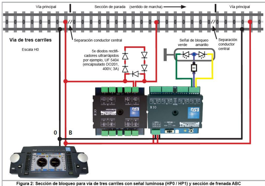
Figura 2: Sección de bloqueo para vía de tres carriles con señal luminosa (HP0 / HP1) y sección de frenada ABC
