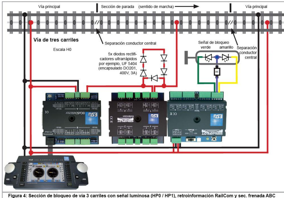
Figura 4: Sección de bloqueo de vía 3 carriles con señal luminosa (HP0 / HP1), retroinformación RailCom y sec. frenada ABC
